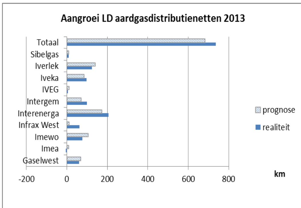
Figuur 10 Realiteit versus prognose aangroei LD net in 2013
