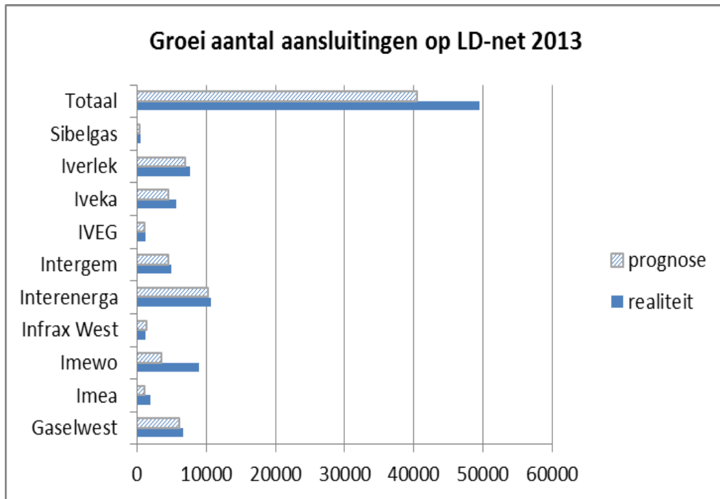
Figuur 11 Realiteit versus prognose aangroei aansluitingen in 2013
